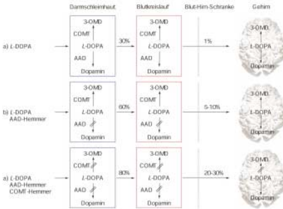
Abb. 2: L-Dopa wird von den Enzymen Aromatische Aminosäure-Decarboxylase (AAD) und Catechol-O-Methyltransferase (COMT) abgebaut bzw. umgewandelt. Werden beide Enzyme gehemmt, gelangen bis zu 30% des Wirkstoffs L-Dopa ins Gehirn.
