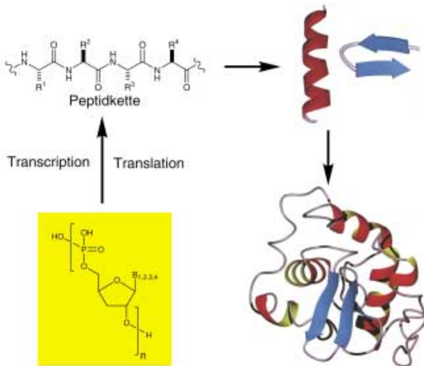
Abb. 2: Vielfalt der natürlichen Proteinwelt: Nach dem Bauplan der DNS («Erbsubstanz») werden die 20 ( R^1, R^2, R^3 \dots verschieden) proteinogenen \alpha -Aminosäuren (NH neben C=O) zu Peptiden (kurze Ketten) bzw. Proteinen (lange Ketten) aneinander gereiht. Schon bei einer Kette aus zehn Aminosäuren (10mer) gibt es 20^{10} ( = 10^{13} oder zehn Trillionen) mögliche verschiedene Sequenzen. Die Ketten falten sich zur «endgültigen» Struktur, wobei es von jedem 10mer wiederum eine Milliarde ( = 10^9 ) verschiedene mögliche räumliche Anordnungen gibt. Die Tertiärstruktur der gefalteten Proteine besteht aus Helices, Faltblättern, Schleifen, ungeordneten Aminosäure-Sequenzen und Disulfid-Brücken. Mehrere Proteine können sich zu grösseren Gebilden zusammenlagern. Durch so genannte postribosomale Modifikationen wie die Anlagerung von Oligosacchariden («Zucker») oder die Phosphatierung wird die Funktion von Proteinen häufig erst ermöglicht.
