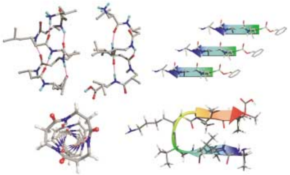
Abb. 1: Einblick in neue Welten: Molekülmodelle von \beta -Peptid-Strukturen, die in Lösung (kernresonanzspektroskopisch) oder im festen Zustand (durch Röntgen-Beugungsmethoden) nachgewiesen wurden: eine links- und eine rechtsgängige Helix, ein paralleles Faltblatt, eine Schleife mit antiparallelem Faltblatt und ein Stapel (im Uhrzeigersinn, beginnend oben links).
