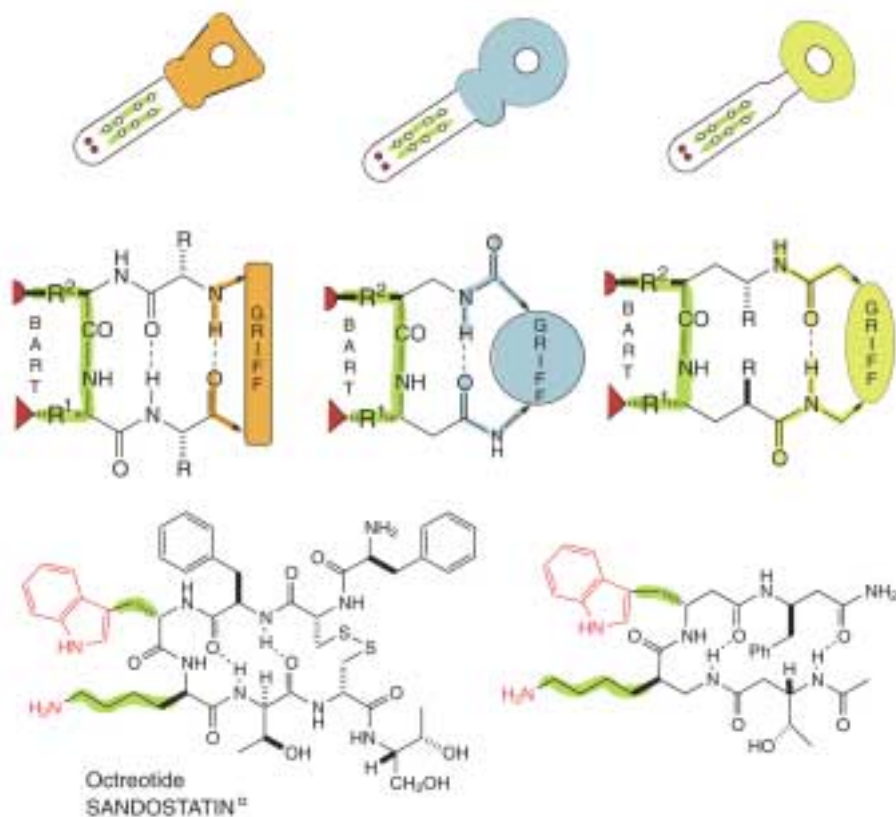
Abb. 4: Nachahmung von \alpha -Peptiden durch \beta - und \gamma -Peptide. Wie Schlüssel mit verschiedenen Griffen, aber identischem Bart dieselbe Tür öffnen (oben), so können \alpha -, \beta - und \gamma -peptidische Schleifen trotz verschiedener Rückgrate (Mitte) an dasselbe Rezeptorprotein andocken, also physiologisch die gleiche Wirksamkeit besitzen. Beispiel: die starke Bindung eines einfachen \beta -Tetra-peptids (Formel unten rechts) an einen der Somatostatin-Rezeptoren, an welche auch das \alpha -peptidische Sandostatin (unten links) bindet. Somatostatin ist ein Säugetier-Peptidhormon, welches wichtige Körperfunktionen reguliert (vgl. zum Beispiel auch das Insulin).
