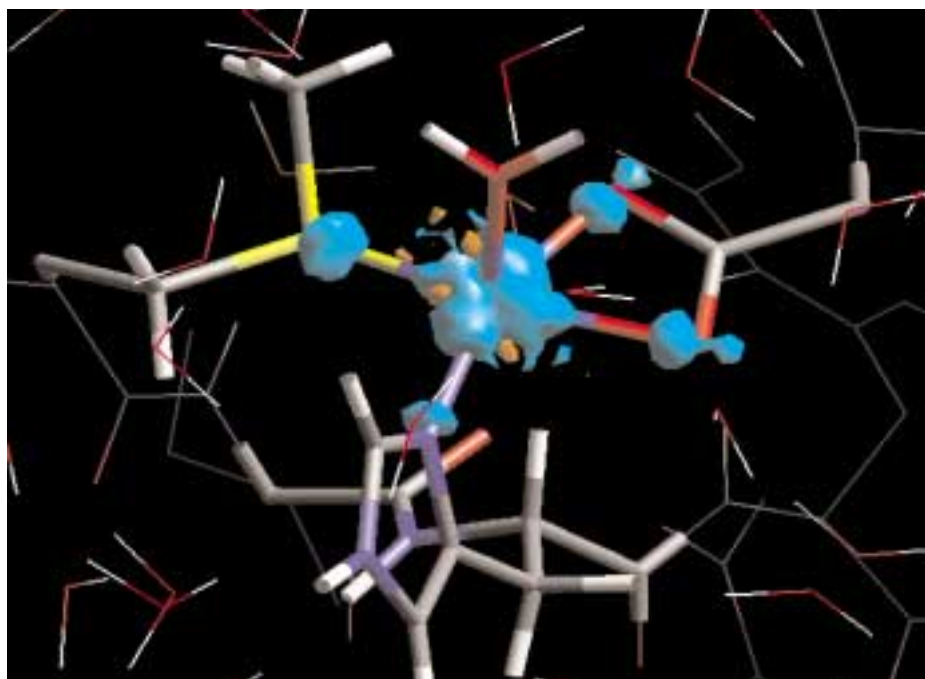
Abb. 4: Mögliche Kupferionen-Bindungsstellen im Prionenprotein von Mäusen.
