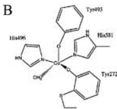
Abb. 3: Das Enzym Galaktose Oxidase (GOase) (A) mit seinem aktiven Zentrum (B). Eine synthetische biomimetische Verbindung von GOase (C).
