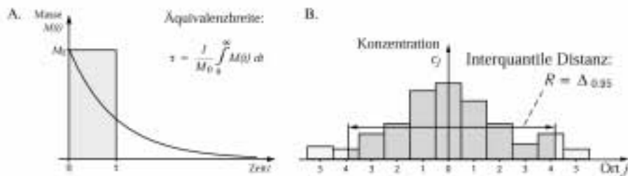
Abb. 3: Persistenz \tau (A) und Reichweite R (B) von Chemikalien in der Umwelt.
