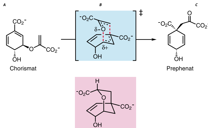
Abb. 1: Die Umlagerung von Chorismat zu Prephenat. Die Reaktion geht über einen kompakten Übergangszustand (blaues Kästchen) vorstatten, indem eine C-O-Bindung und eine C-C-Bindung fast gleichzeitig gebrochen bzw. gebildet werden (gestrichelte rote Linien). Konformationell eingeschränkte Verbindungen (rosa Kästchen), welche den Übergangszustand imitieren, sind wirkungsvolle Inhibitoren für Chorismatmutase-Enzyme und wurden auch für die Herstellung von katalytischen Antikörpern erfolgreich eingesetzt.
