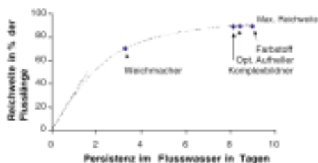
Abb. 4: Reichweite und Aufenthaltszeit im Flusswasser für ausgewählte Chemikalien gemäss dem Flussmodell (nach Beck et al. 2000).
