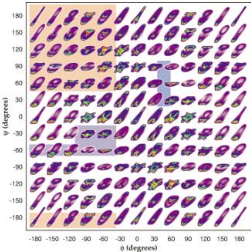
Abb. 4: Berechnete zweidimensionale NMR-Spektren für 169 verschiedene Kombinationen der Winkel \phi und \psi . Die rot unterlegten Winkelbereiche entsprechen dem Beta-Faltblatt-Bereich, die dunkelblau unterlegten der Alpha-Helix und die hellblau unterlegten einer linkshändigen Alpha-Helix. (Spektren: J. van Beek)
