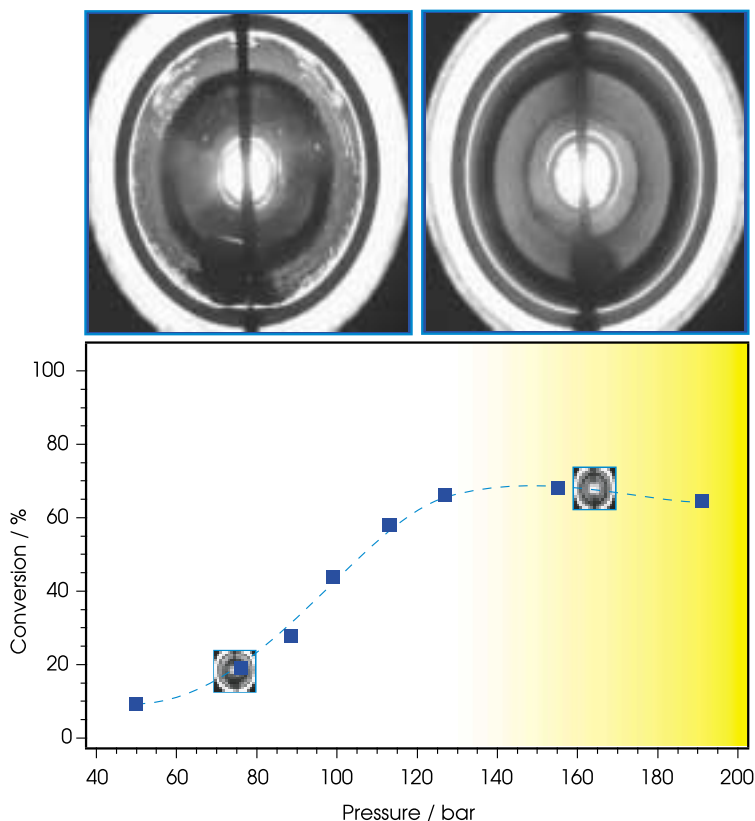
Abb. 5: Hydrierung von Phenylacetylen: Umsatz als Funktion des Drucks bei 55°C. Die Löslichkeit des flüssigen Eduktgemisches hängt vom Druck ab. Erst bei etwa 135 bar erreicht der Reaktorinhalt das Einphasengebiet (gelb).
