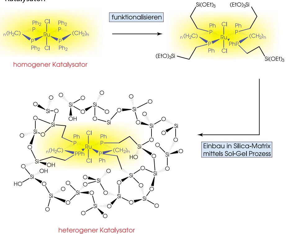
Abb 2: N,N -Dimethylformamid kann durch Einsatz von Ruthenium-Komplex-Katalysatoren ( n=1,3 ) aus Kohlendioxid produziert werden. Mit der Immobilisierung der Komplexe in ein Silica-Netzwerk können leicht wiederverwendbare heterogene Hybrid-Katalysatoren gewonnen werden.
