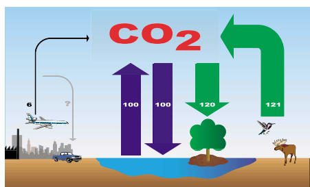
Abb. 1: Die vereinfachten Kohlendioxid-Kreisläufe der Atmosphäre. Die Zahlen stehen für 10^9 t Kohlenstoff pro Jahr.
