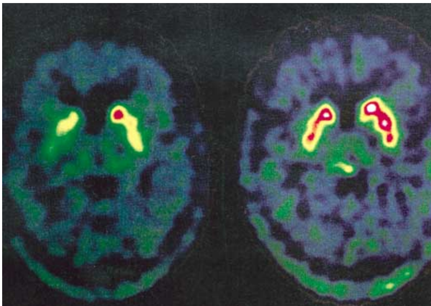
Abb. 1: L-Dopa ist ein wichtiger Wirkstoff in der Behandlung von Parkinson-Patienten. Damit genügend davon ins Hirn gelangt, muss verhindert werden, dass L-Dopa bereits im Körper umgewandelt wird. PET-Abbildungen des Gehirns eines Parkinson-Patienten, dem radioaktiv markiertes L-Dopa intravenös verabreicht wurde. Links: ohne COMT-Hemmstoff. Rechts: nach Verabreichung des COMT-Hemmstoffs Entecapone zeigt sich deutlich eine grössere Anreicherung von L-Dopa in bestimmten Hirnregionen. [Copyright: Zeitschrift «Neurology»]
