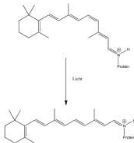
Abb. 2: Fotoinduzierte Cis-trans-Isomerisierung von Retinal
