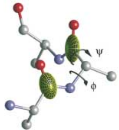
Abb. 3: Definition der beiden Winkel \phi und \psi in einer Aminosäure. Sind diese beiden Winkel für jede Aminosäure bekannt, ist die Struktur des «Rückgrats» des Proteins vollständig bestimmt.
