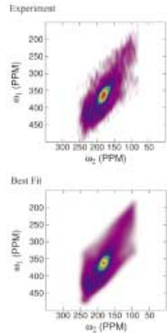
Abb. 5: Experimentelles zweidimensionales NMR-Spektrum von Alanin-markierter Seide der wilden Seidenraupe Samia cynthia ricini und bester Fit. (Spektren: J. van Beek)
