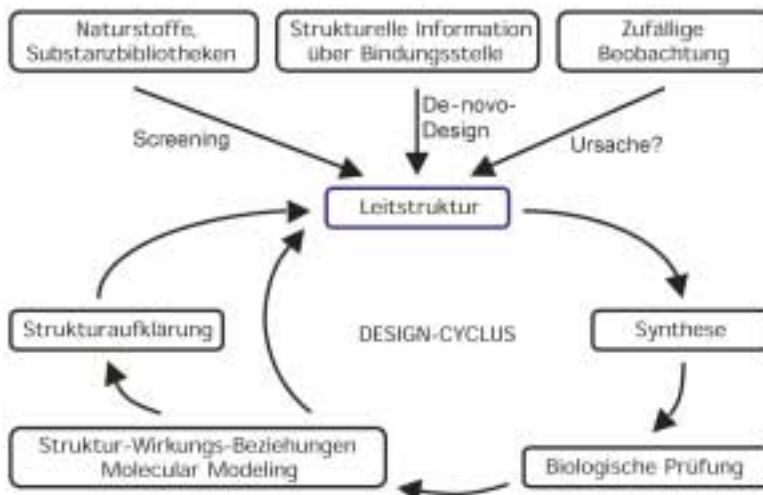
Abb. 3: Der iterative Prozess des strukturbasierten Wirkstoffdesigns: Der Design-Zyklus muss in den meisten Fällen mehrfach durchlaufen werden, bevor eine Struktur in weitere Entwicklungsstufen der Arzneimittelforschung gelangt.
