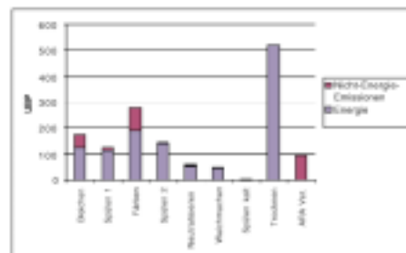
Abb. 2: Ökobilanz nach UBP für das vollständige (d. h. Energiebereitstellung und sonstige Prozessschritte) und für das reduzierte (d. h. nur Energiebereitstellung) Ökoinventar (Funktionelle Einheit: Veredlungsschritt für ein rotes Baumwoll-T-Shirt [250 g]).
