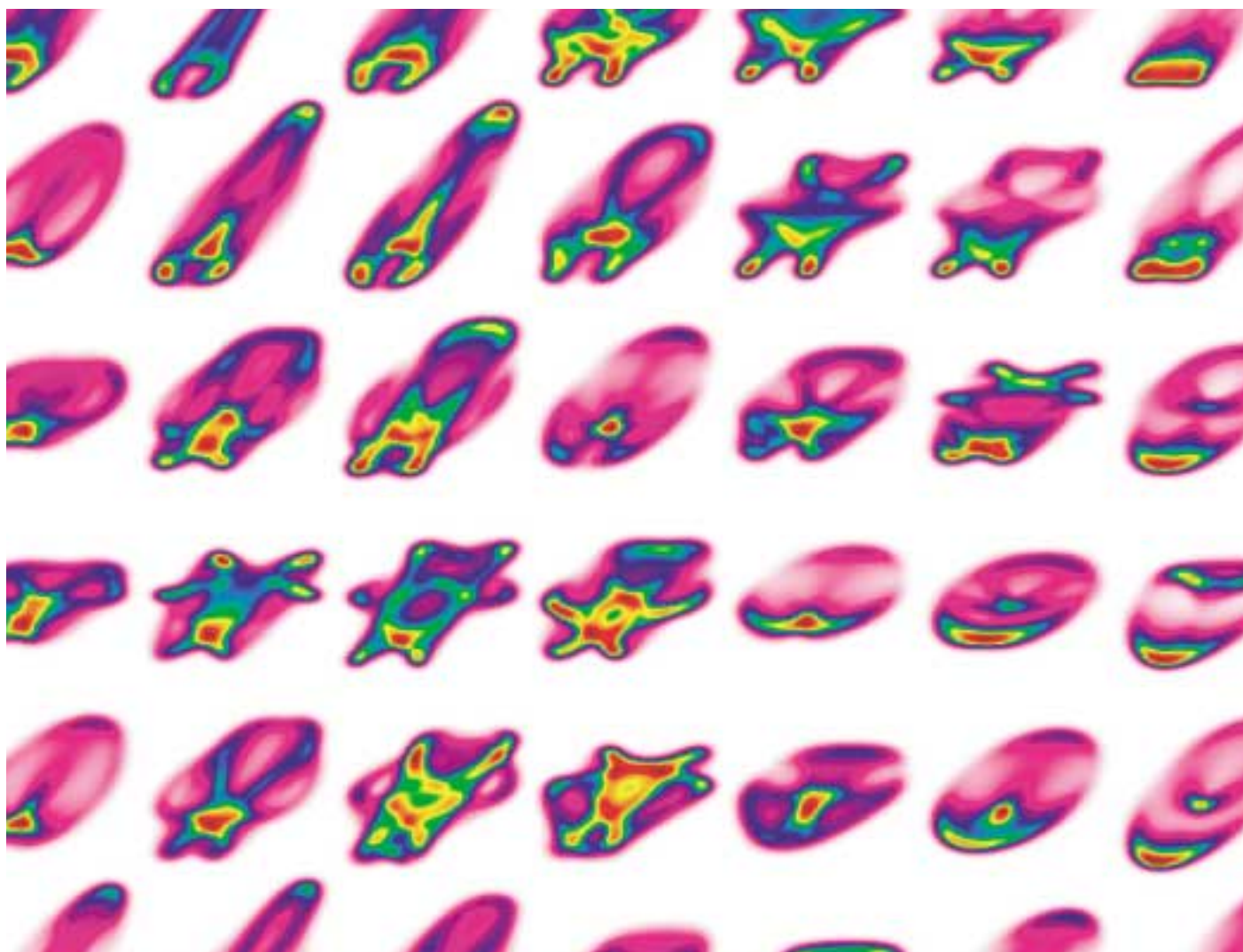
Abb. 1: NMR-Spektren – Detail aus Abbildung 4, Seite 38.
