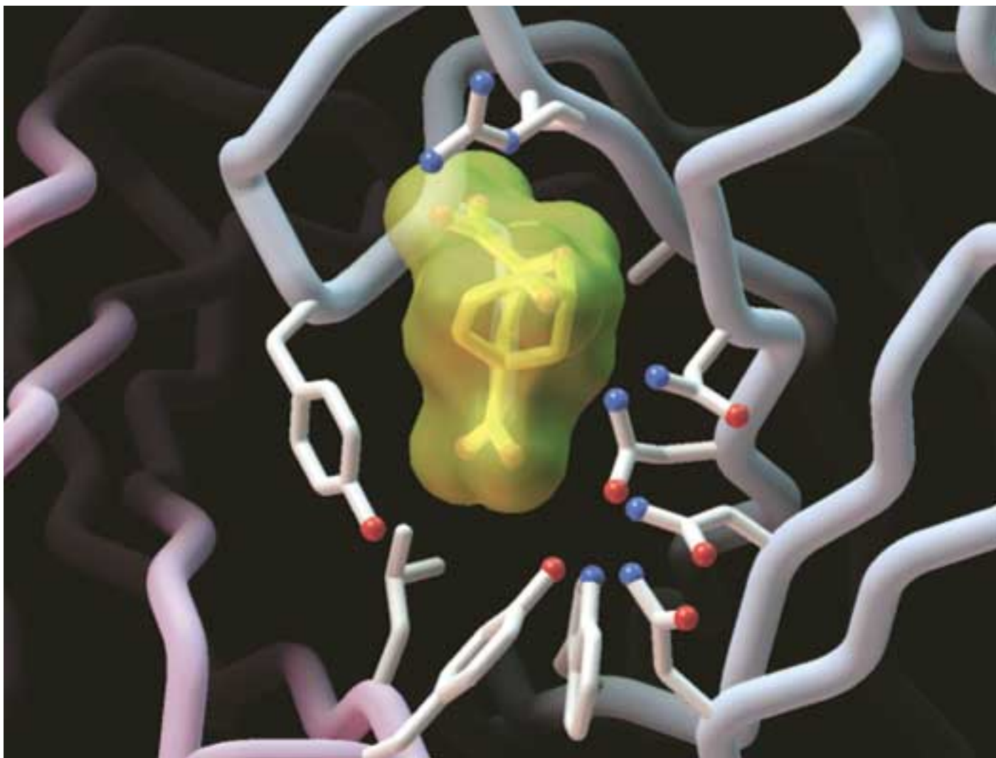
Abb. 2: Die aktive Tasche des katalytischen Antikörpers 1F7, der unter Verwendung des Übergangszustands-Analogons aus Abbildung 1 (als gelbes Stabmodell mit einer molekularen Oberfläche gezeichnet) erzeugt wurde. Der Antikörper nutzt die Seitenketten vieler verschiedener Aminosäuren aus, um das Analogon spezifisch zu erkennen. (Bilderstellung: Michael Pique)
