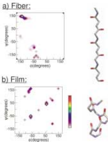
Abb. 6: Wahrscheinlichkeitsverteilung der Torsionswinkel \phi und \psi für die Alanine in der Seide der wilden Seidenraupe Samia cynthia ricini . a) Verteilung für einen Seidenfaden. Die Sekundärstruktur ist hauptsächlich Beta-Faltblatt; b) Verteilung für einen künstlich hergestellten Film aus derselben Seide. Hier ist die Sekundärstruktur vorwiegend alpha-helical. Adaptiert aus: J. van Beek et al., «Nature», (2000). «Solid-State NMR determination of the secondary structure of Samia Cynthia Ricini silk.» «Nature» 405: 1077–1079.
