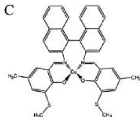
Abb. 3: Das Enzym Galaktose Oxidase (GOase) (A) mit seinem aktiven Zentrum (B). Eine synthetische biomimetische Verbindung von GOase (C).
