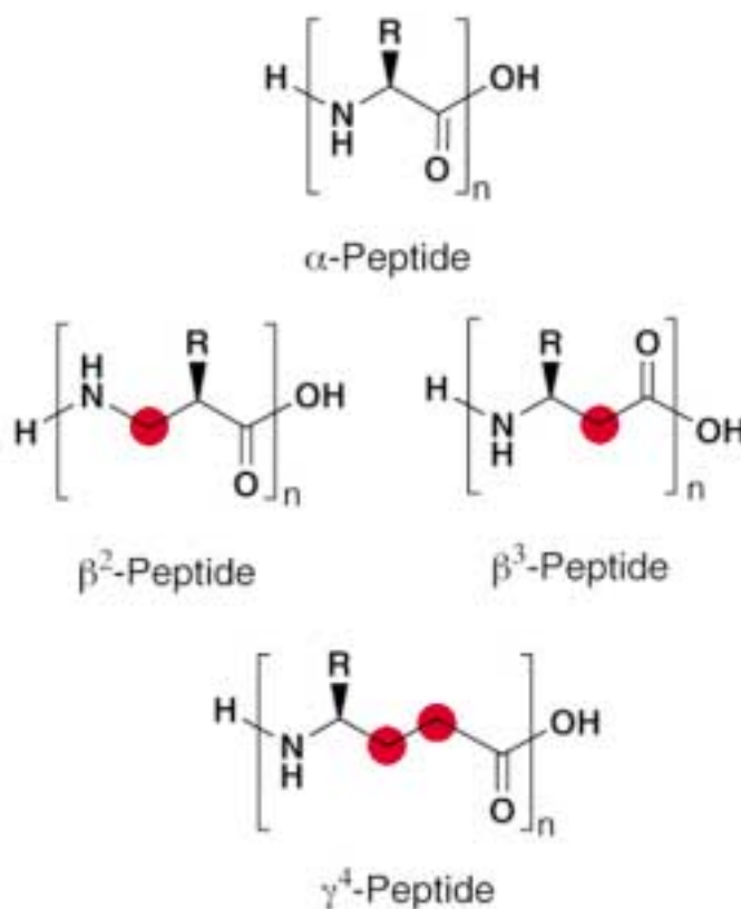
Abb. 3: Vergleich der Strukturformeln von \alpha -Peptiden (und Proteinen) mit denen von \beta - und \gamma -Peptiden, welche sich durch Einschieben einer bzw. zweier \text{CH}_2 -Gruppen («Homologisierung») in jeden Aminosäure-Baustein ergeben. Die hochgestellten Zahlen ( \beta^2 , \beta^3 , \gamma^4 ) geben an, in welcher Position der entsprechenden Aminosäure die Seitenkette R steht. Das Suffix n gibt an, wie viele Bausteine die Peptidkette enthält.
