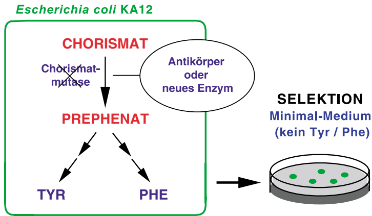
Abb. 3: Ein Selektionssystem für Chorismatmutase-Aktivität. E.-coli-Zellen ohne endogene Chorismatmutase sind in Abwesenheit von Tyrosin (Tyr) und Phenylalanin (Phe) unfähig zu wachsen. Neu eingeführte Gene, welche für Proteine mit Chorismatmutase-Aktivität kodieren, werden auf Grund ihrer Fähigkeit, den genetischen Defekt aufzuheben und damit den Zellen das Wachstum zu gestatten, selektiert.
