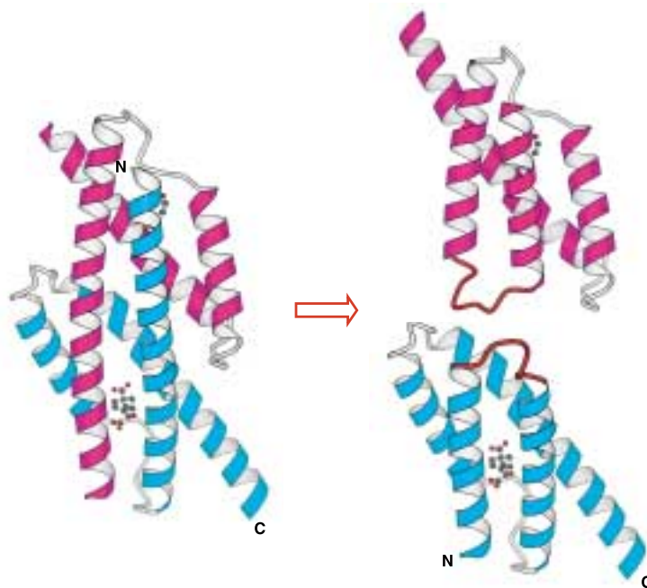
Abb. 4: Topologische Verwandlung eines dimeren Chorismatmutase-Enzyms in ein Monomer. Das Einfügen einer flexiblen Schleife in die Helix, die das Dimer durchspannt, erlaubt es der N-terminalen Hälfte der Helix, sich auf sich selbst zurückzuklappen, dadurch das andere Polypeptid zu ersetzen und so einen funktionellen Katalysator mit 4-Helixbündelstruktur zu bilden.
