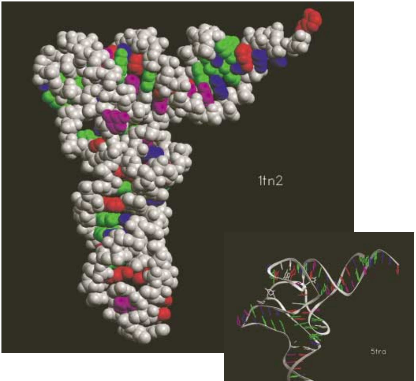
Der Stoff der Xeragon AG: RNA-Moleküle dreidimensional dargestellt.
