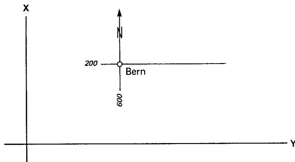
Figur 3-6 Schweizerisches Landeskoordinatensystem
