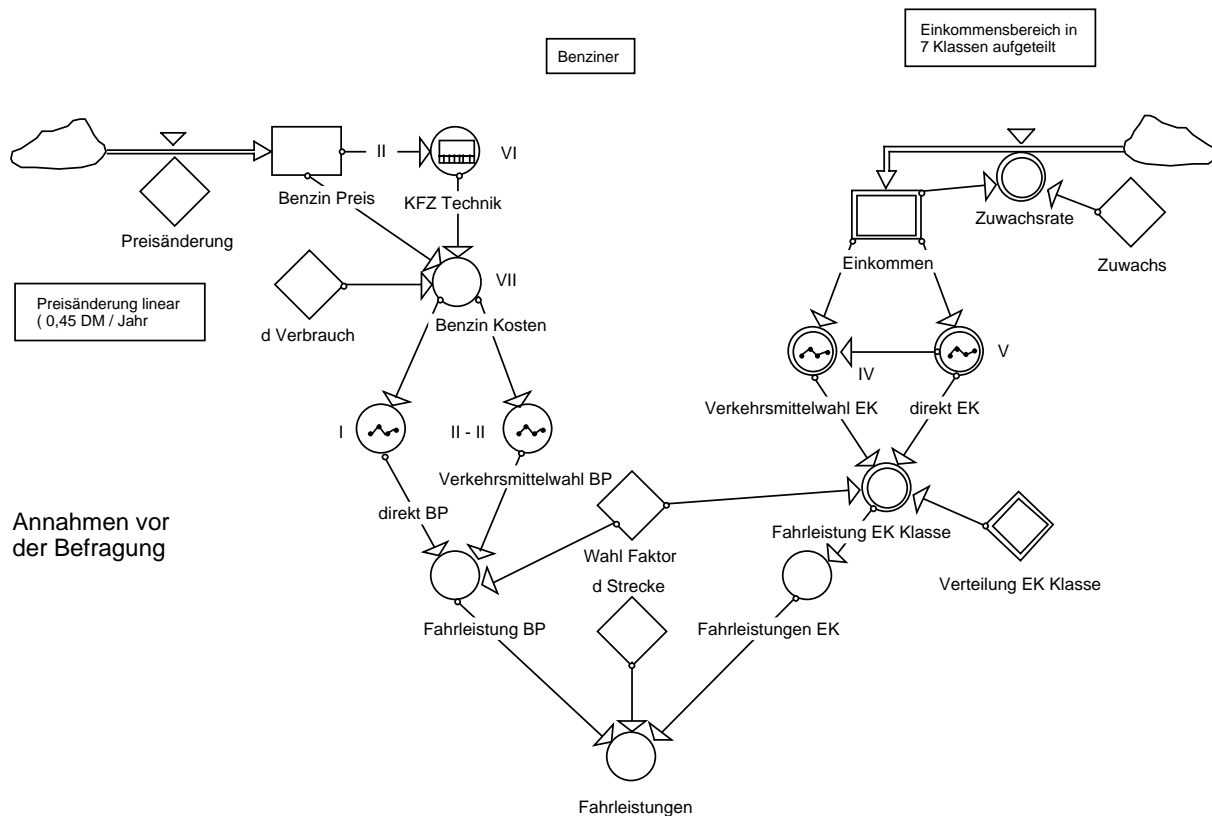
Abbildung 2 Flussdiagramm
