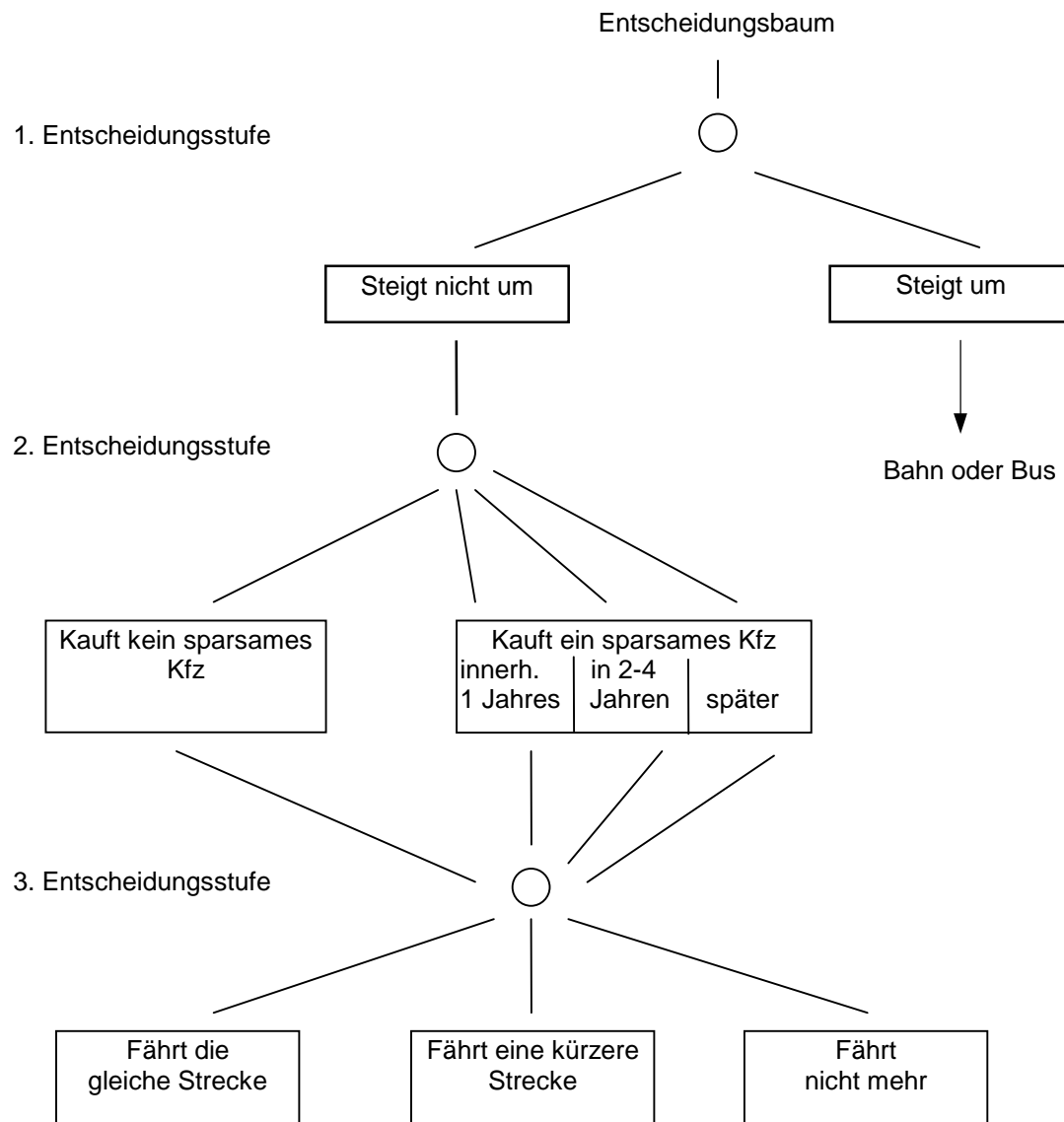
Abbildung 3 Unterstellter Entscheidungsbaum
