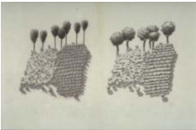
Dickung
