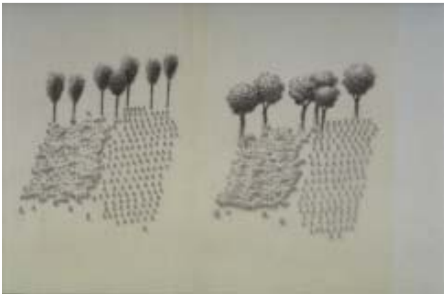
Jungwuchs
