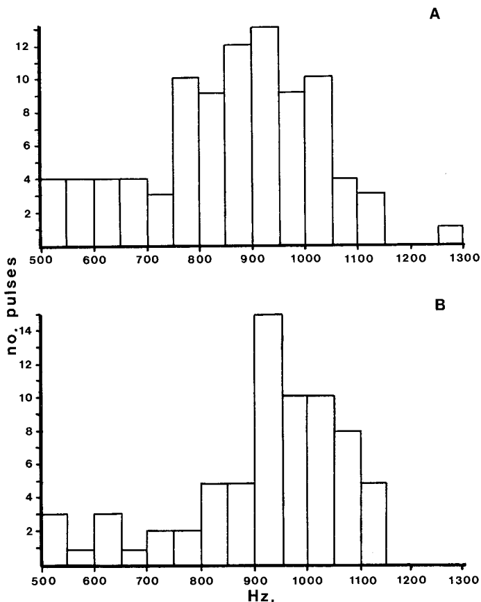
Fig. 8. Histograms of sample fundamental frequencies. A: S. bipunctata . B: S. borealis .
