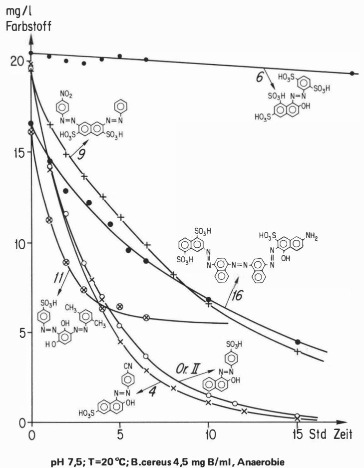
Abb. 2: Entfärbung von Azofarbstoffen durch B. cereus unter sauerstofffreien Bedingungen.
