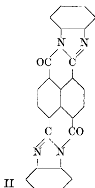
II trans-Form des Naphthoylen-di-benzimidazols Indanthrenbrillantorange GR
