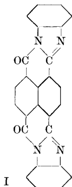
I cis-Form des Naphthoylen-di-benzimidazols blauroter nicht interessanter Küpenfarbstoff
