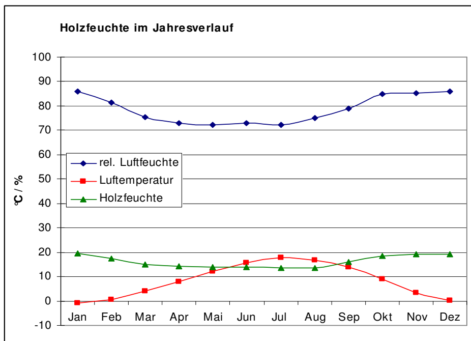
Abbildung 26 Holzgleichsfeuchte von Aussenbauteilen unter dem Einfluss von relativer Luftfeuchte und Temperatur. Die Klimadaten stammen von MeteoSchweiz (Normwerte 1961-1990; Wetterstation Zürich-Kloten)
