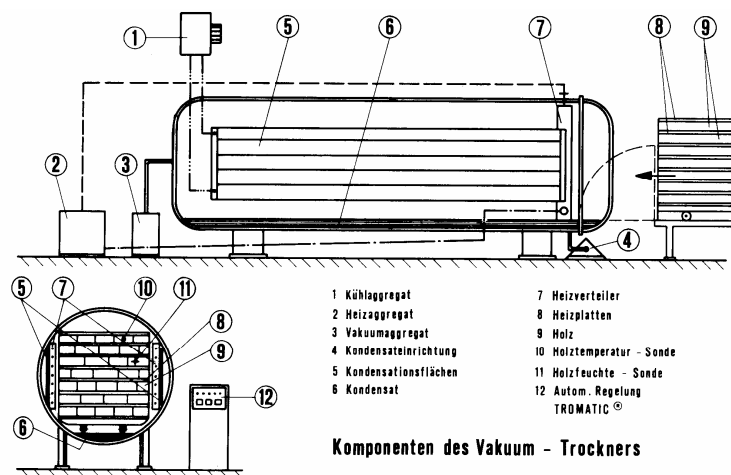
Abbildung 18 Vakuumtrockner (Bollmann)
